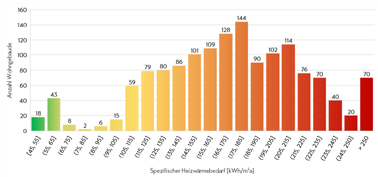
Abbildung 12: Energieeffizienz des Gebäudebestandes in der Gemeinde Schönau am Königssee
