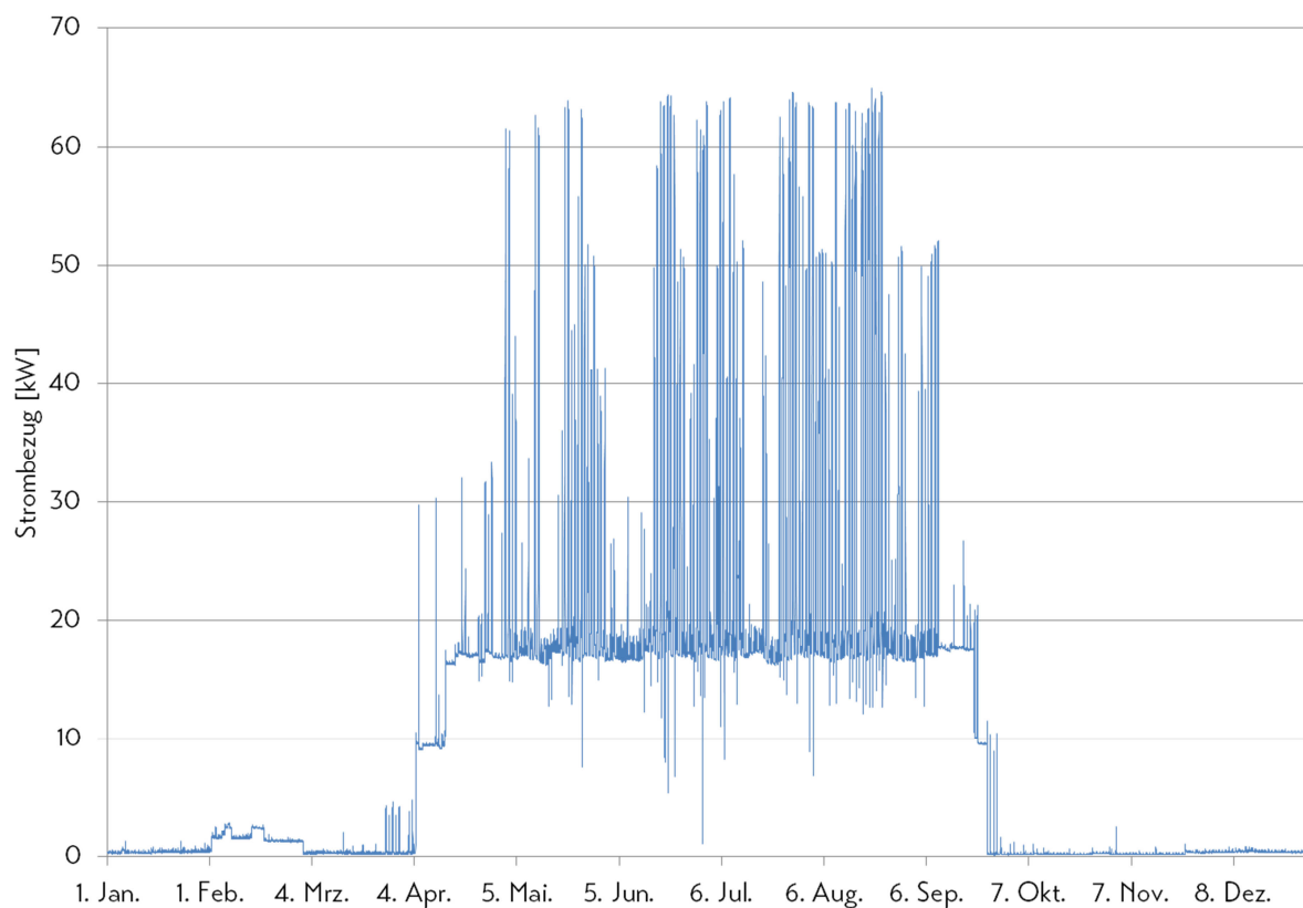
Abbildung 31: Simulierter elektrischer Lastgang des Schornbads
