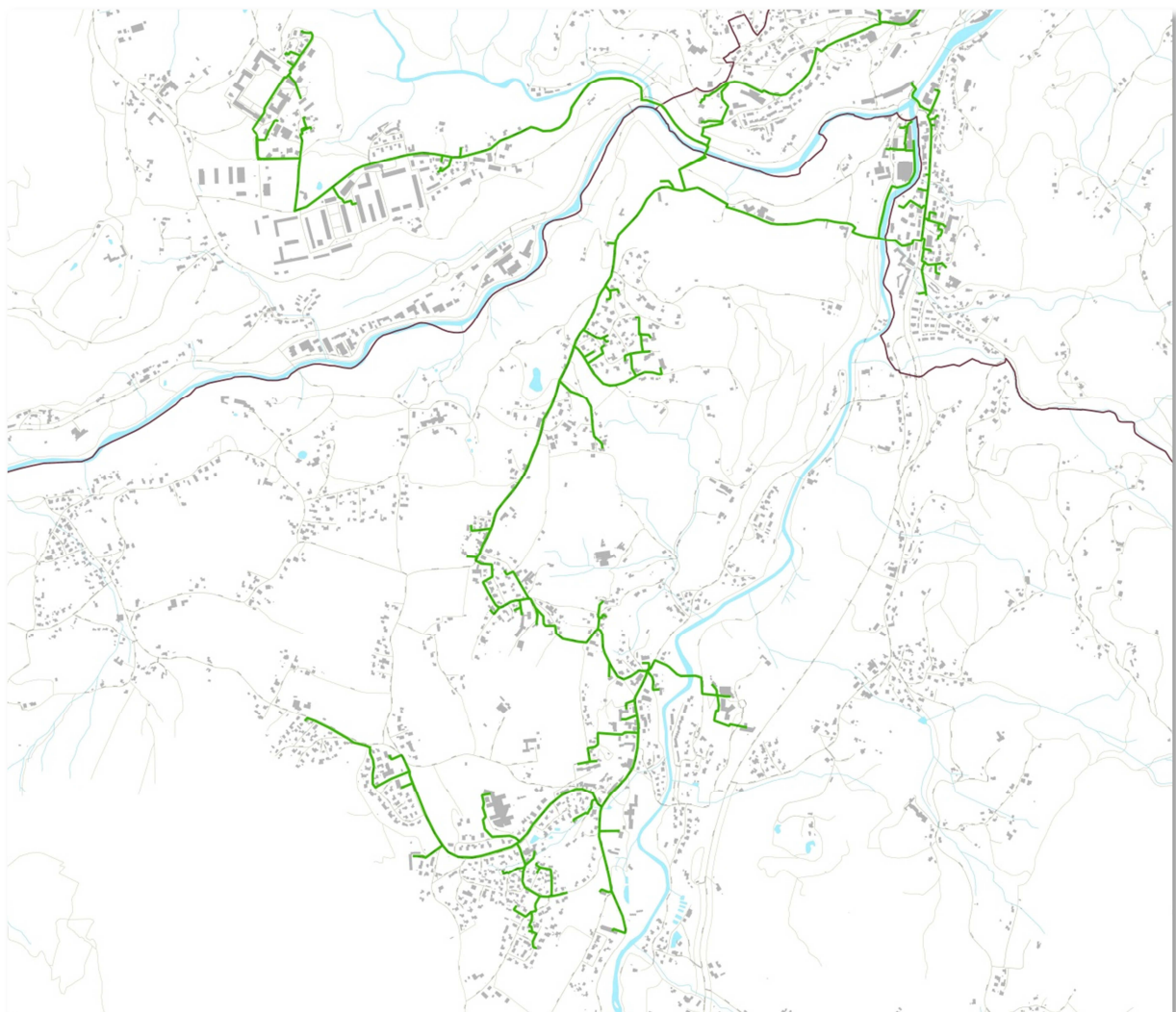
Abbildung 11: Fernwärmeversorgung der Bioenergie Berchtesgadener Land im Gemeindegebiet Schönau a. Königssee (Stand 2014)
