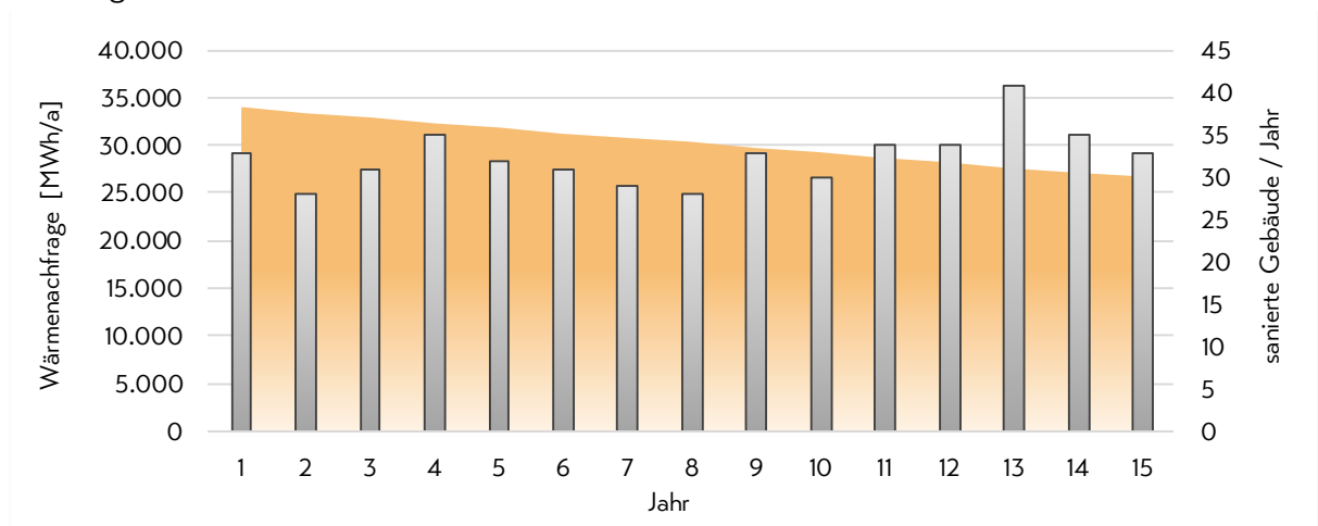
Abbildung 14: Sanierungspotenzial Wohngebäude in der Gemeinde Schönau am Königssee
