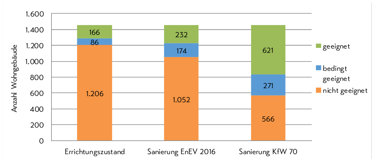
Abbildung 22: Versorgungspotenzial durch Erdwärmesonden in der Gemeinde Schönau am Königssee
