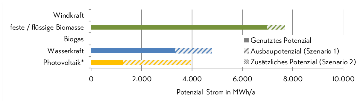
Abbildung 15: Genutzte Potenziale und Ausbaupotenziale erneuerbarer Energien zur Stromerzeugung
