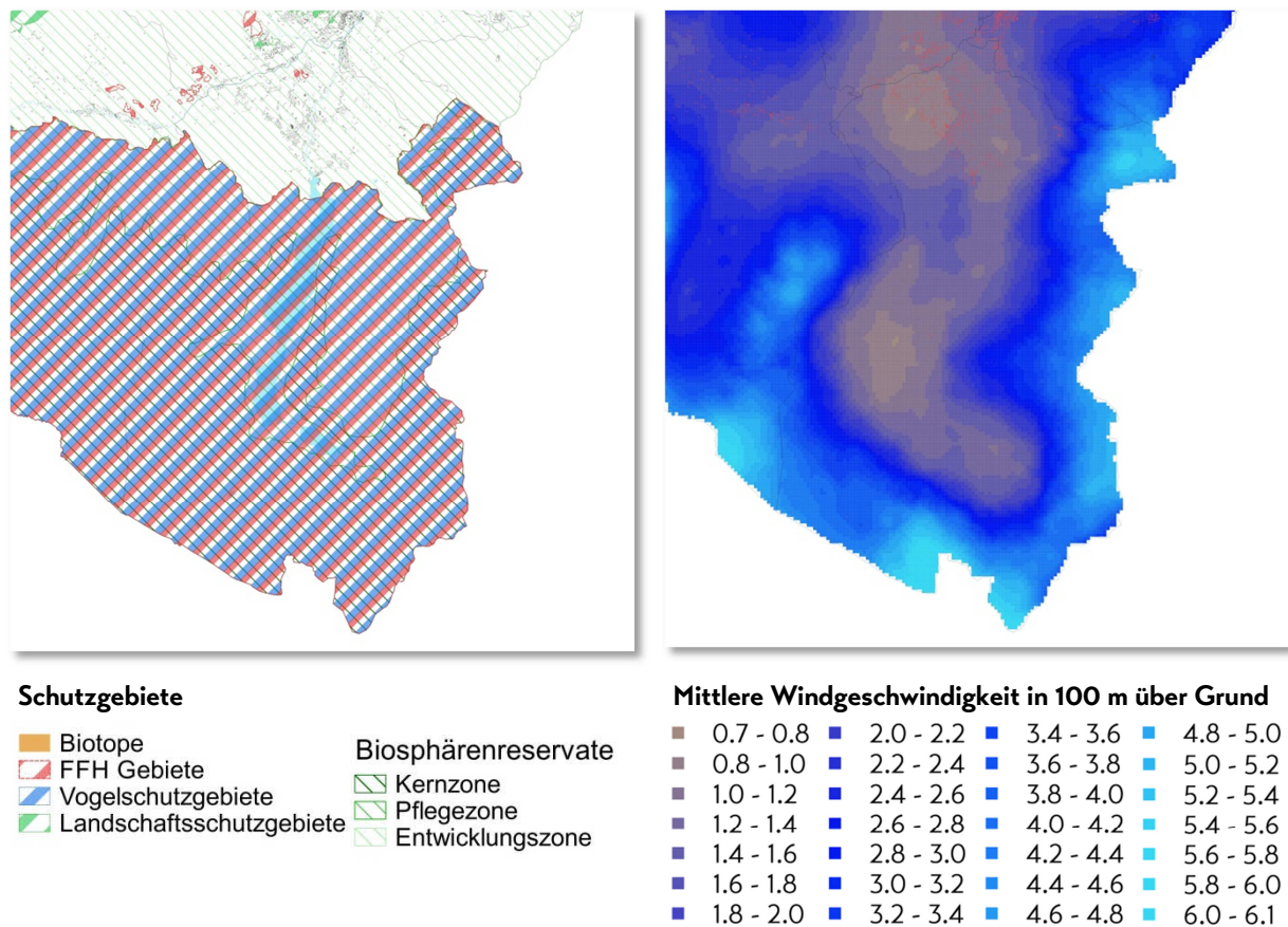
Abbildung 24: Schutzgebietskartierung (links) und mittlere Jahreswindgeschwindigkeit in 100 m ü. G. (rechts)
