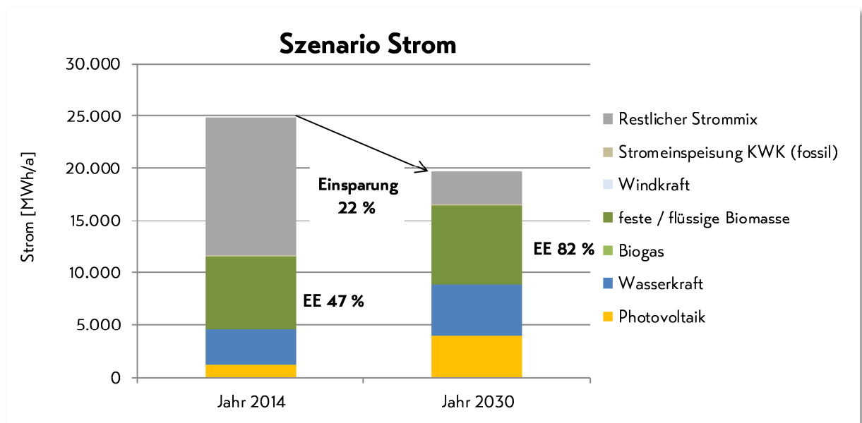
Abbildung 27: Szenario Strom
